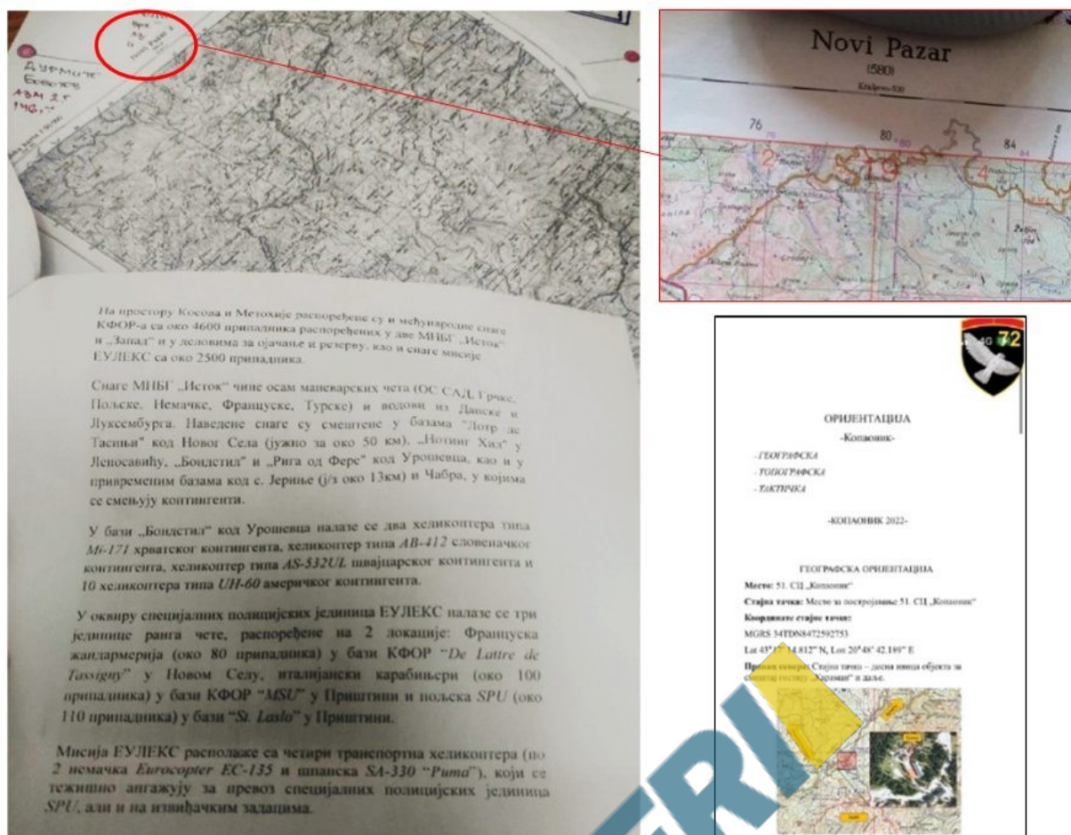
Figure 28: Kopaonik 2022
